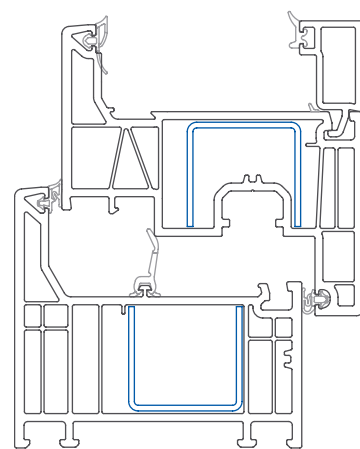
Elegante - поверхні профілів каскадом. Масштаб 1:2
