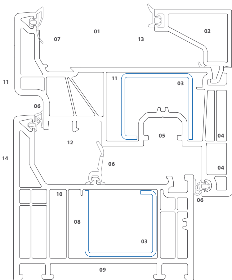
Elegante - поверхні профілів в рівень. Масштаб 1:1
