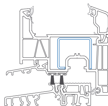
Elegante з теплим алюмінієвим порогом та закругленою рейкою - Масштаб 1:2
