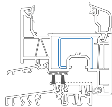
Elegante Balkontürschwelle mit schräger Glasleiste · Abb.: 1:2
