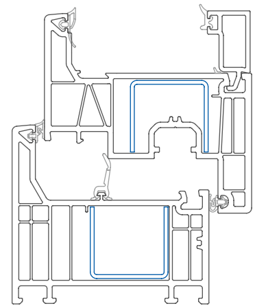
Elegante flächenversetzt mit eckiger Glasleiste · Abb.: 1:2
