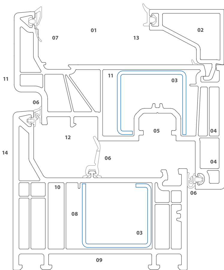
Elegante profil zlicowany Skala 1:1
